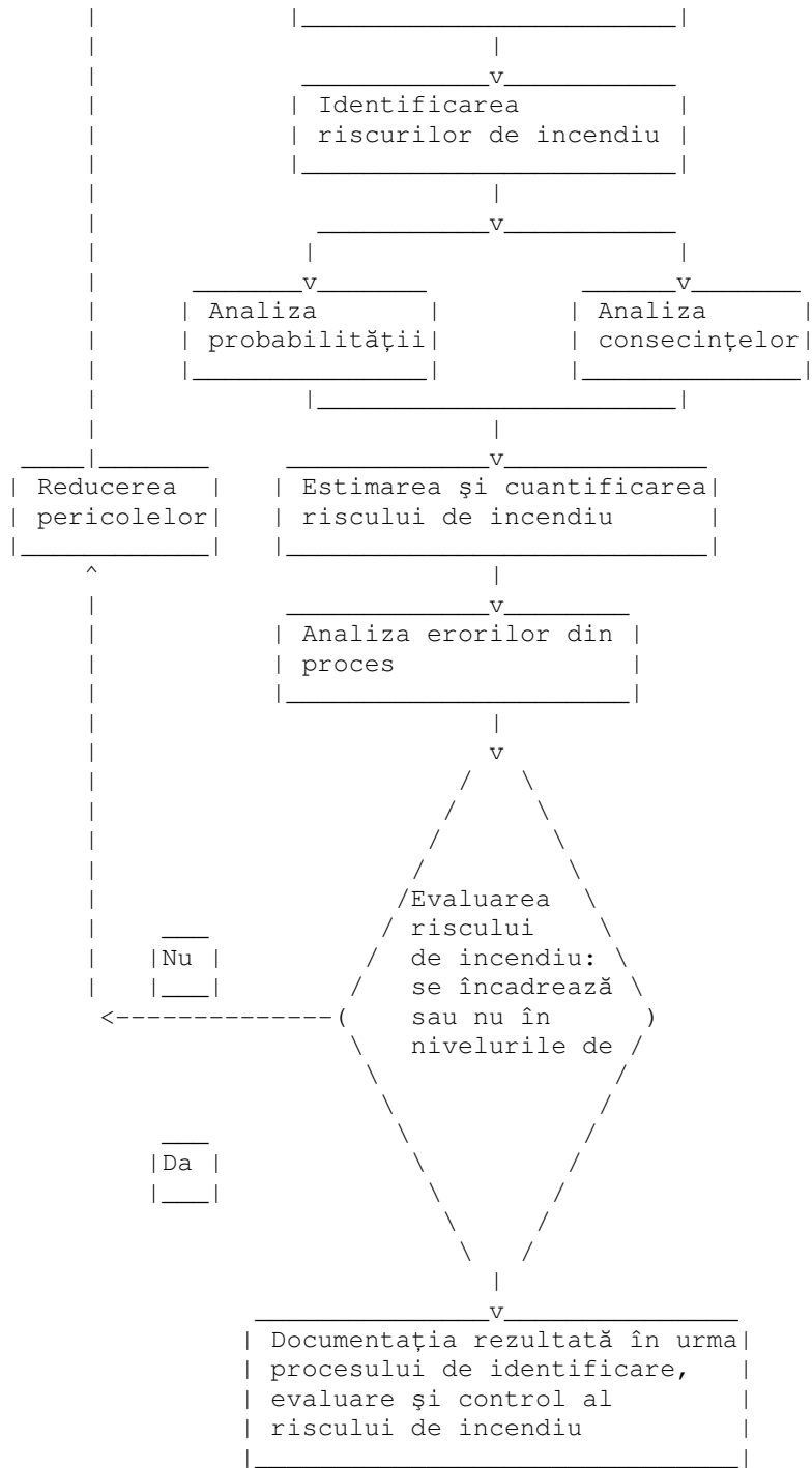
Schema logică de management al riscurilor de incendiu în faza de proiectare
